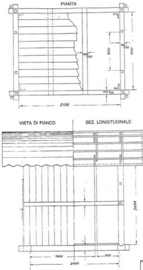
TIPO DI CASOTTO SMONTABILE PER Kg. 500 DI ESPLOSIVI
