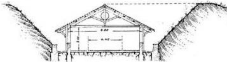
SEZ. TRASVERSALE
