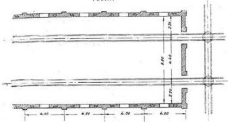
TIPO DI BARACCA PER MATERIALI ESPLOSIVI PIANTA
