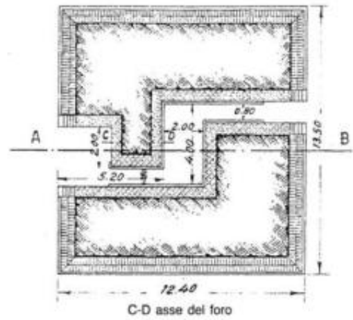
TIPO DI CELLA BLINDATA PIANTA
